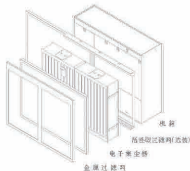
KJFF3700-2603 结构示意图
