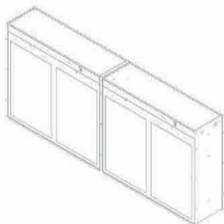
KJFF3700-2603 模块化扩容示意图
