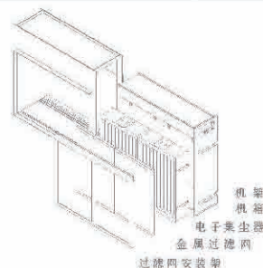
KJFF3700-2612 结构示意图
